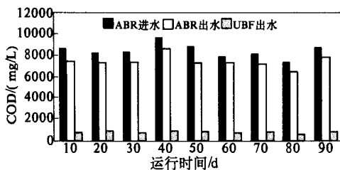
图 5 COD 在两相厌氧处理系统中的变化 Fig. 5 Variations of COD in the two phase anaerobic digestion system
