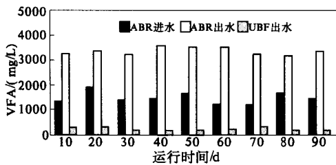
图 4 VFA 在两相厌氧处理系统中的变化 Fig. 4 Variations of VFA in the two phase anaerobic digestion system
