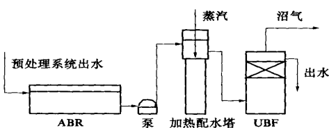
图1 两相厌氧处理抗生素废水的工艺装置
